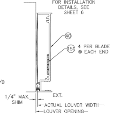
B 3 JAMB DETAIL
