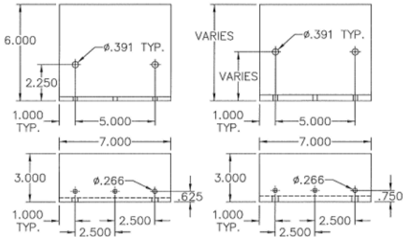
157 3x6x1/4" ALUMINUM
