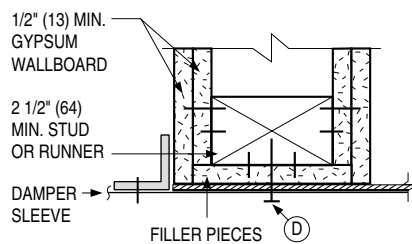
G: Wood Stud Detail
