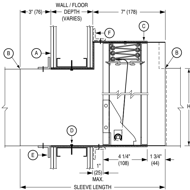
TYPE B VERTICAL MOUNT, (D)0120DOW
