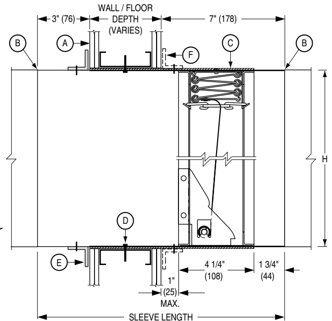
TYPE A VERTICAL MOUNT, (D)0110DOW
