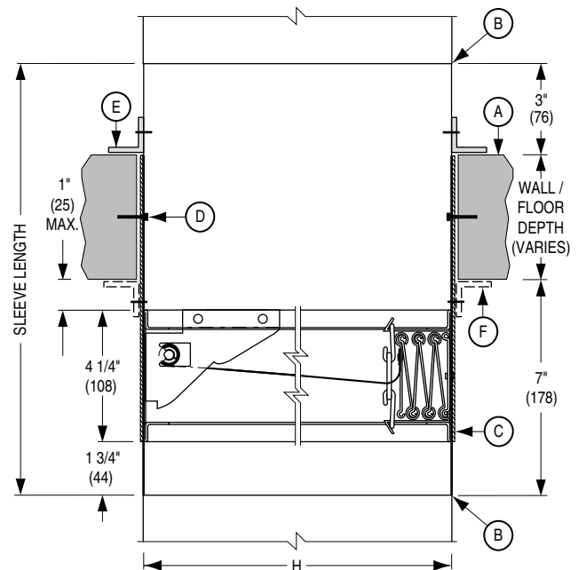
TYPE A HORIZONTAL MOUNT, (D)0110DOW
