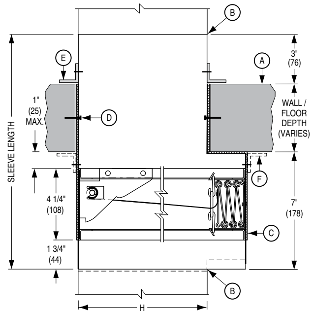
TYPE B HORIZONTAL MOUNT, (D)0120DOW
