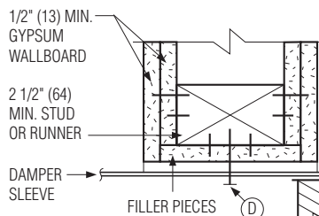
I: Wood Stud Detail
