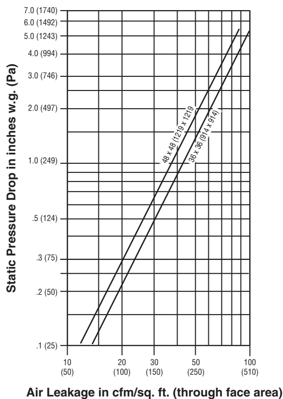
Tested per AMCA standard 500-D, Fig. 5.5.
